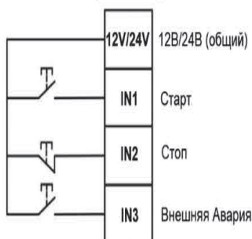
0: Стандартное применение
