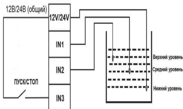
3: Датчик уровня 1
