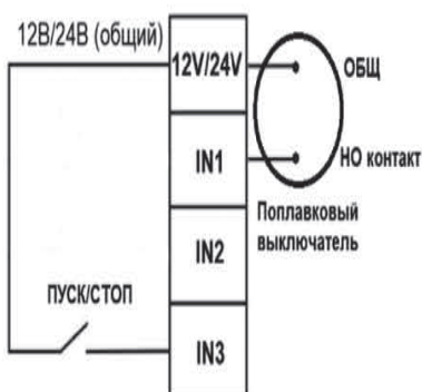
1: Поплавковый выключатель
